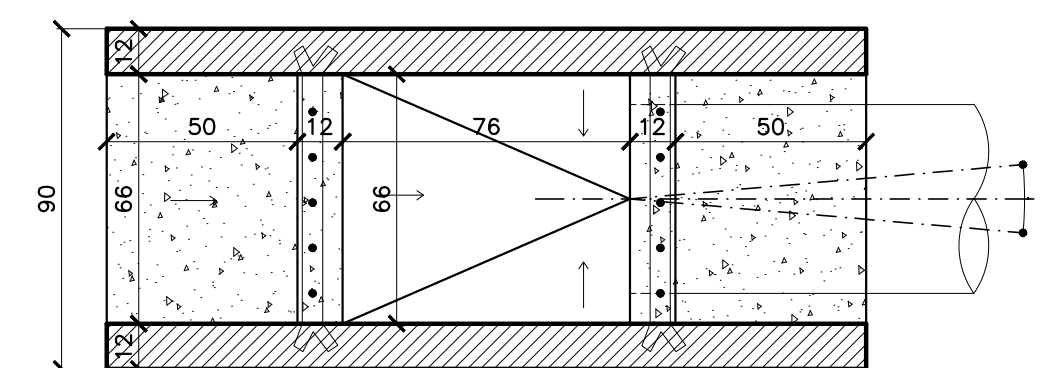
VARIANTE PLANTA DE SALIDA
