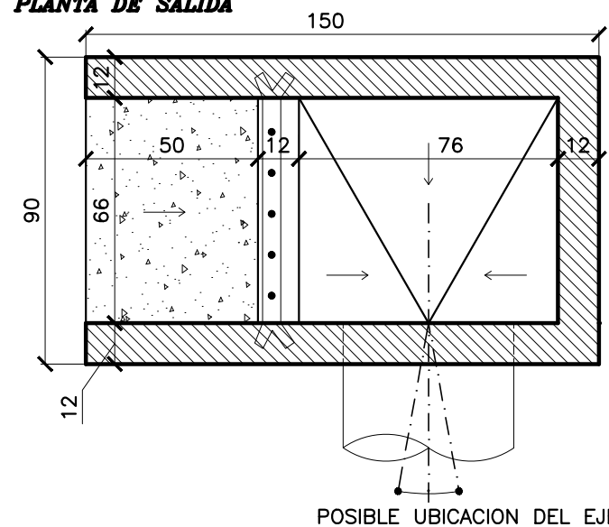
VARIANTE PLANTA DE SALIDA
