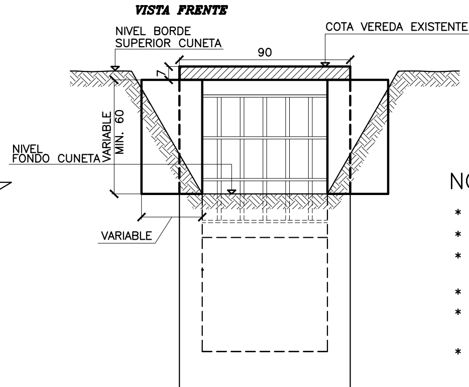
VISTA FRENTE
