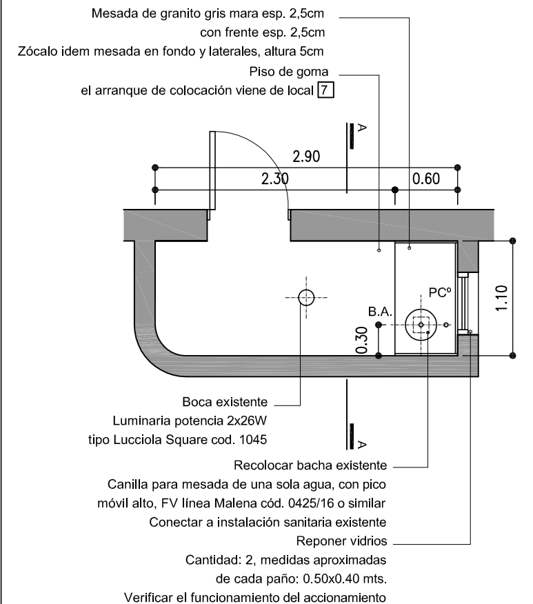
PLANTA OFFICE Esc. 1:50
