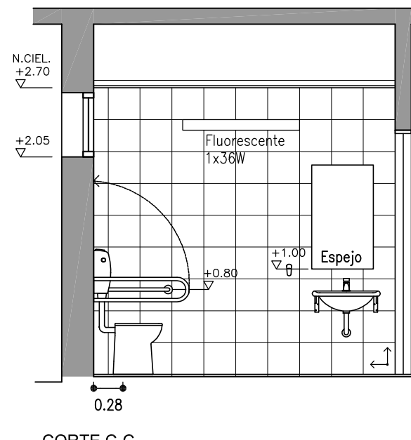
CORTE C-C Esc. 1:50
