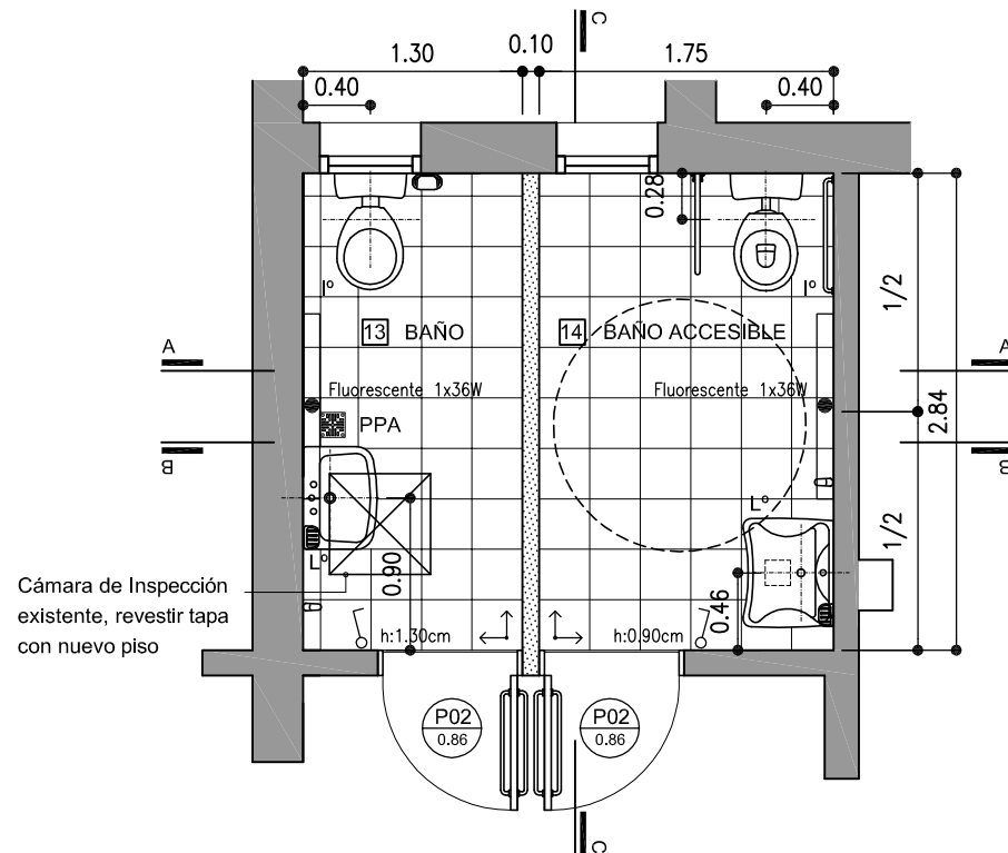
PLANTA DE BAÑOS Esc. 1:50
