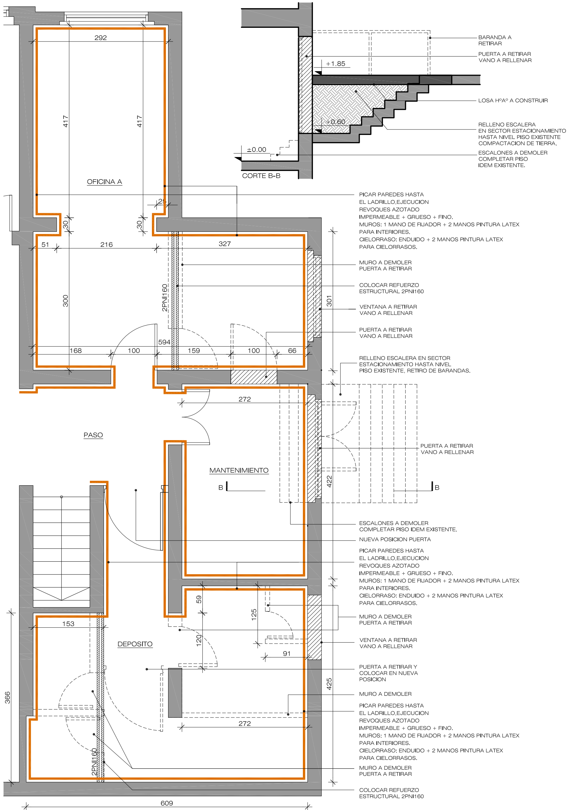
PLANTA SECTOR OFICINA A / DEPÓSITO / MANTENIMIENTO ESCALA 1:50
