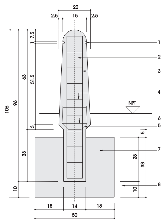
DETALLE CONSTRUCTIVO
