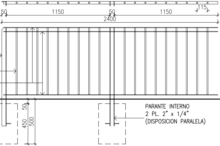
PLANTA
