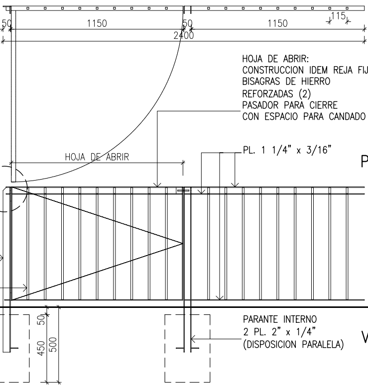
PLANTA
