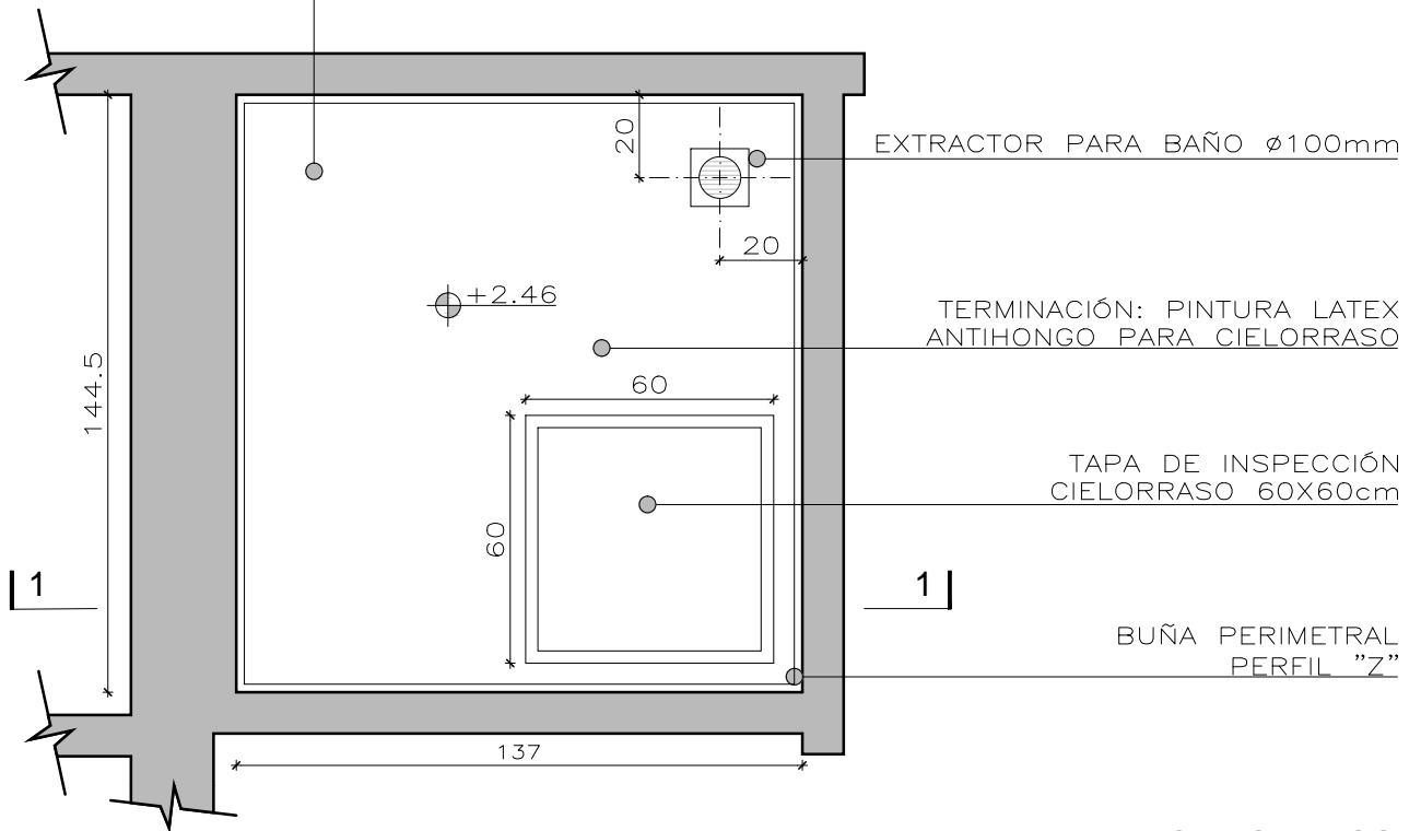
PLANTA CIELORRASO
