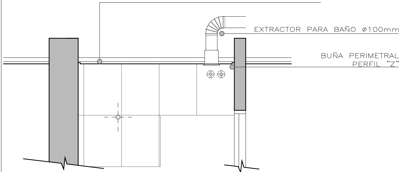
CORTE 1-1 CIELORRASO
